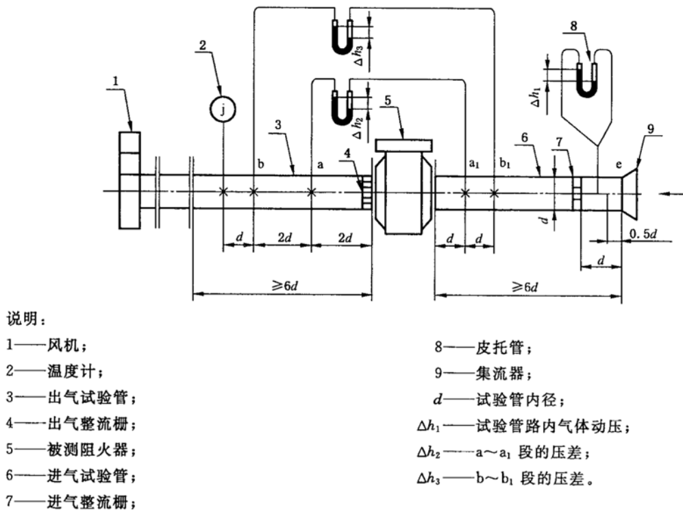
图 3 压力损失和通气量试验装置示意图
