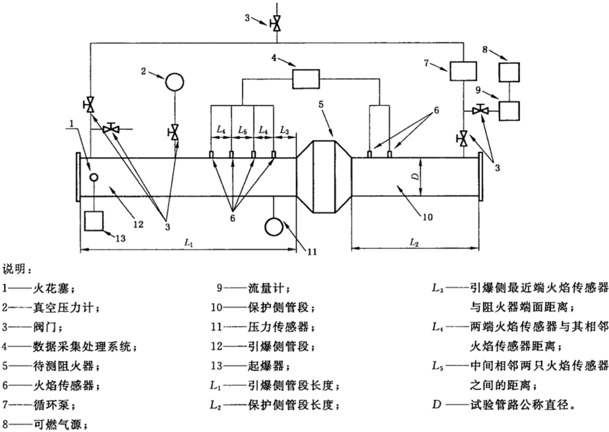
图 1 阻爆试验装置示意图
